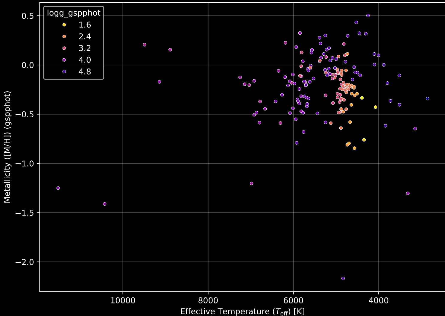
APOGEE DR17 Field: [CVZTILE_091+35_btx] Stellar Population Parameters (n= 189)
